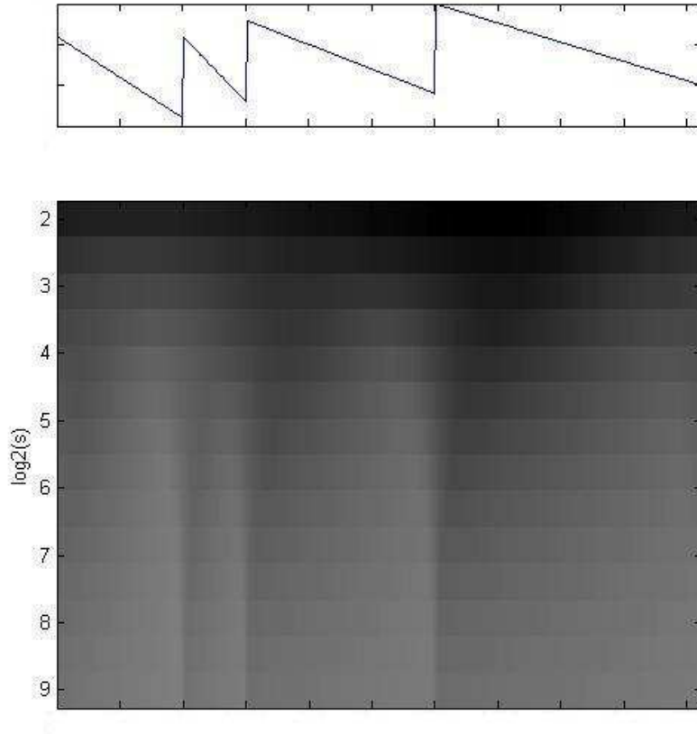
Figure 4. Décomposition en ondelettes d'un signal simulant un processus de réplication de l'ADN chez les mammifères.
